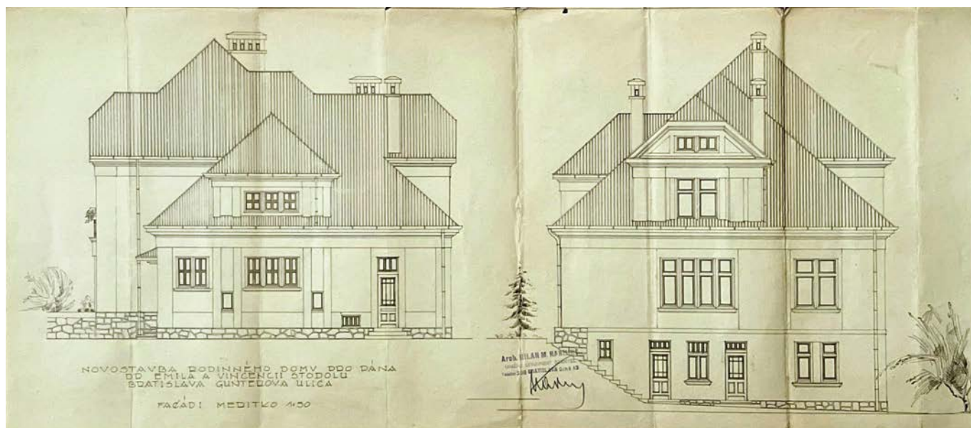
Vila E. Štodolu (M. M. Harminc). Zdroj: Štátny archív v Bratislave, f. Daňová správa v Bratislave. Foto: B. Bartalos, M. Kušnírová.
