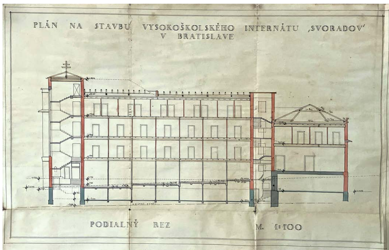
Projekt na stavbu internátu Svoradov (G. Schreiber a F. Florians). Zdroj: Štátny archív v Bratislave, f. Daňová správa v Bratislave. Foto: B. Bartalos, M. Kušnírová.
